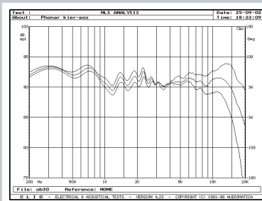
rys. 3a. Zakres 200Hz - 20kHz, na osi głównej i pod kątami 15^\circ i 30^\circ w płaszczyźnie poziomej, pomiar metodą MLS z odległości 1,5 m.
