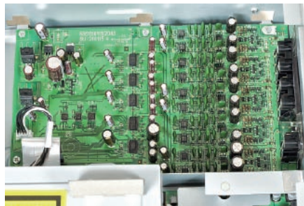
Sekcję audio zbudowano aż z pięciu dwukanałowych torów, a każdy wyposażono w stereofoniczny przetwornik C/A...
