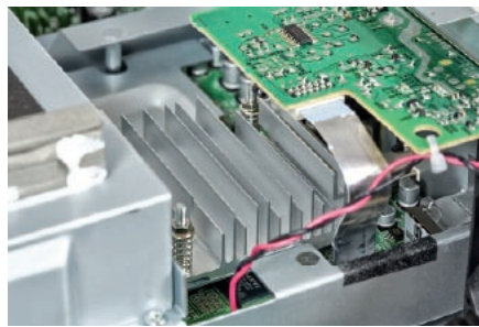
Pod dużym radiatorem ukrywa się bardzo dobry procesor obrazu ABT.
