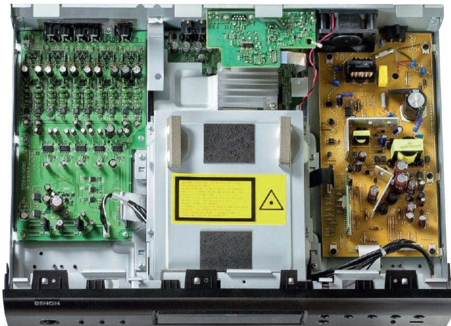
Wszystkie układy podzielono między funkcjonalne moduły.
